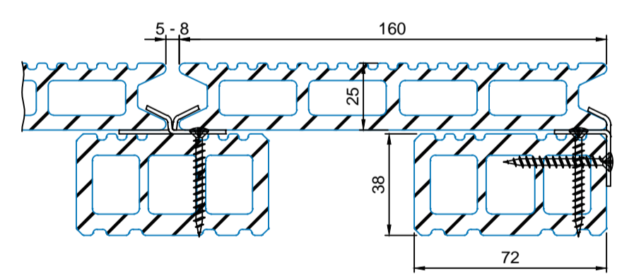
2121 .. Verlängerung (WPC) / 2221 .. Anschlussprofil 63 mm / 2222 .. Trennleiste
