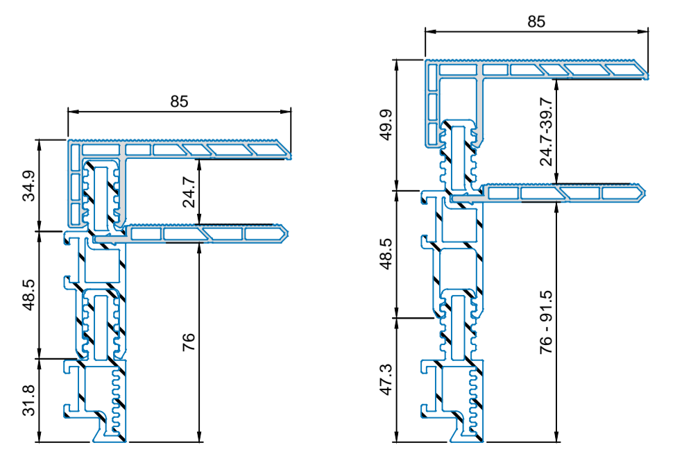
2120 .. Grundprofil (WPC) / 2121 .. Verlängerung (WPC) 2221 .. Anschlussprofil 63 mm / 2222 .. Trennleiste
