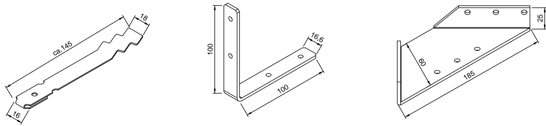
2410 .. Bauklammer 2411 .. Winkel 2415 .. Eckwinkel 120x120x25 mm 2416 .. Eckverbinder 40x40 mm
