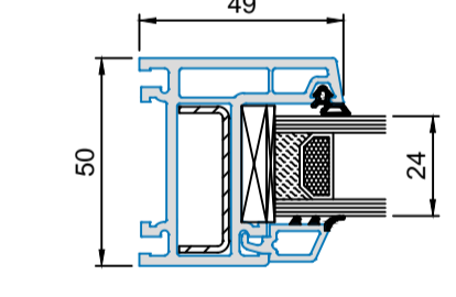
989 .. Rahmen / 990 .. Flügel
