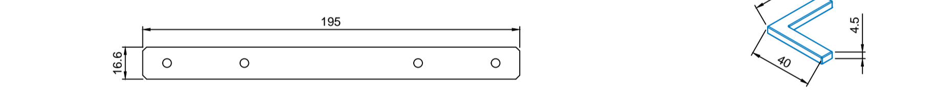
2414 .. Modulverbinder 2416 .. Eckverbinder 40x40 mm
