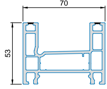
5101 .. Rahmen 70 / 53
