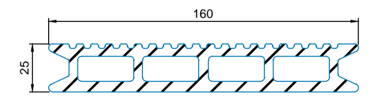
2101 .. WPC - Dielen 74 schokobraun 75 schwarz 76 cedar 77 rotbraun 78 hellgrau
