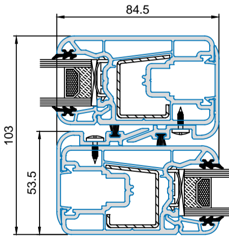
5204 .. Verschlussprofil
