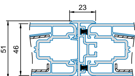
5203 .. Stulpleiste
