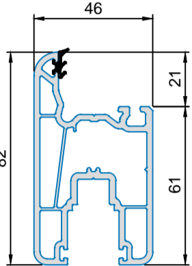
5102 .. Flügel
