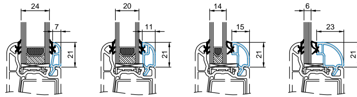
5201 .. Glas 24 mm 5202 .. Glas 20 mm 1203 .. Glas 14 mm 1204 .. Glas 6 mm
