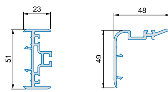
5203 .. Stulpleiste 5204 .. Verschlussprofil
