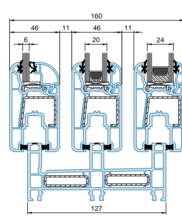
5104 .. Rahmen 70/127 5102 .. Flügel
