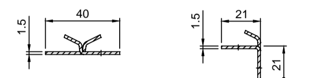
2421 .. Montageklammer Bodendielen 2422 .. Randklammer Bodendielen
