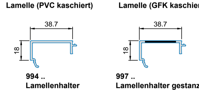
994 .. Lamellenhalter 997 .. Lamellenhalter gestanzt 5652 .. Stahlverstärkung 5653 .. Stahlverstärkung 988 .. Stahlverstärkung
