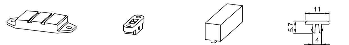
5305 .. Dichtklotz 00 weiss 02 olivbraun 06 cremeweiss 5306 .. Laufrolle (Moskito) 5307 .. Distanzklotz 6215 .. Nutabdeckungsprofil
