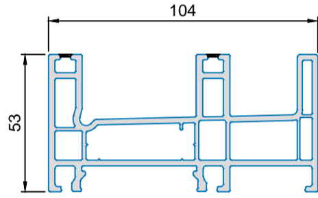
5103 .. Rahmen 70 / 104
