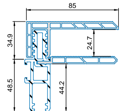
2120 .. Grundprofil (WPC) / 2121 .. Verlängerung (WPC) 2221 .. Anschlussprofil 63 mm / 2222 .. Trennleiste
