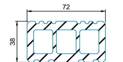
2201 .. Unterkonstruktion 38 mm
