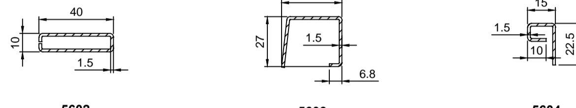
5602 .. 5603 .. 5604 ..
