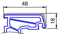
8701 .. Dualschale Flügel 79
