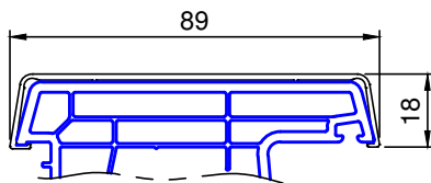
8705 .. Dualschale Stulp breit
