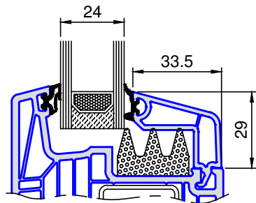
8212 .. Glasleiste Festverglasung Glas 24mm
