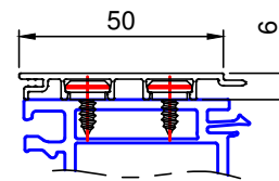
8706 .. Dualschale Verbreiterung 50/80 mm
