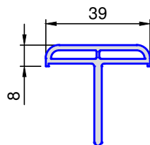
1219 .. Verglasungsprofil 1
