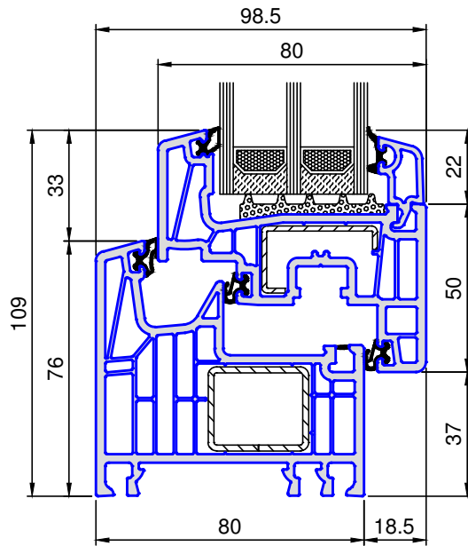
8101 .. Rahmen 76
