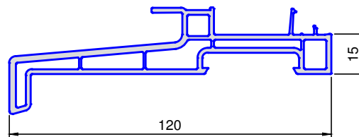
8222 .. Fensterbank 120x15
