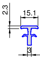
7225 .. Verbindungsstück
