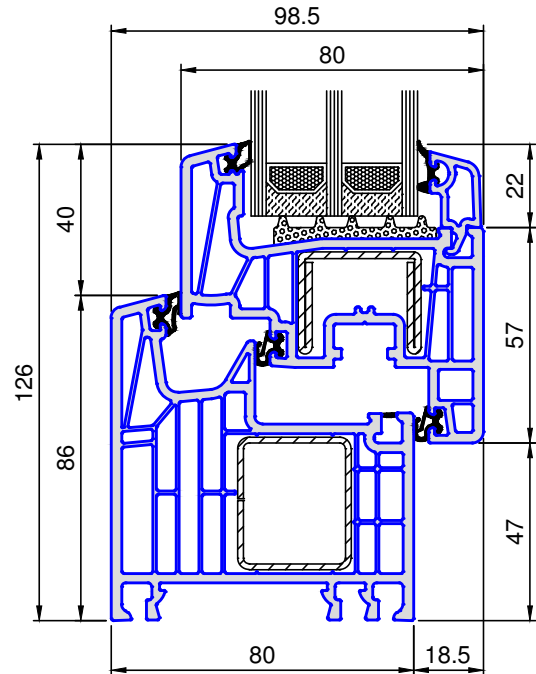
8102 .. Rahmen 86
