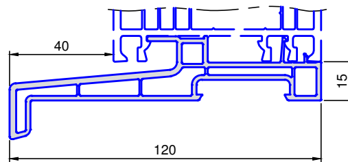
8222 .. Fensterbank 120x15
