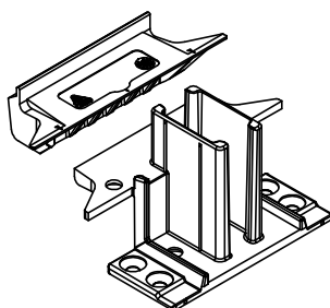
8308 .. Verbinder für Pfosten
