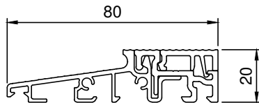
8401 .. Schwelle Alu EV1 20 / 70 mm
