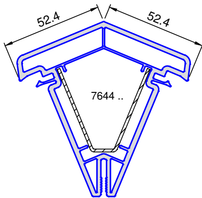
7208 .. Eckprofil 135°
