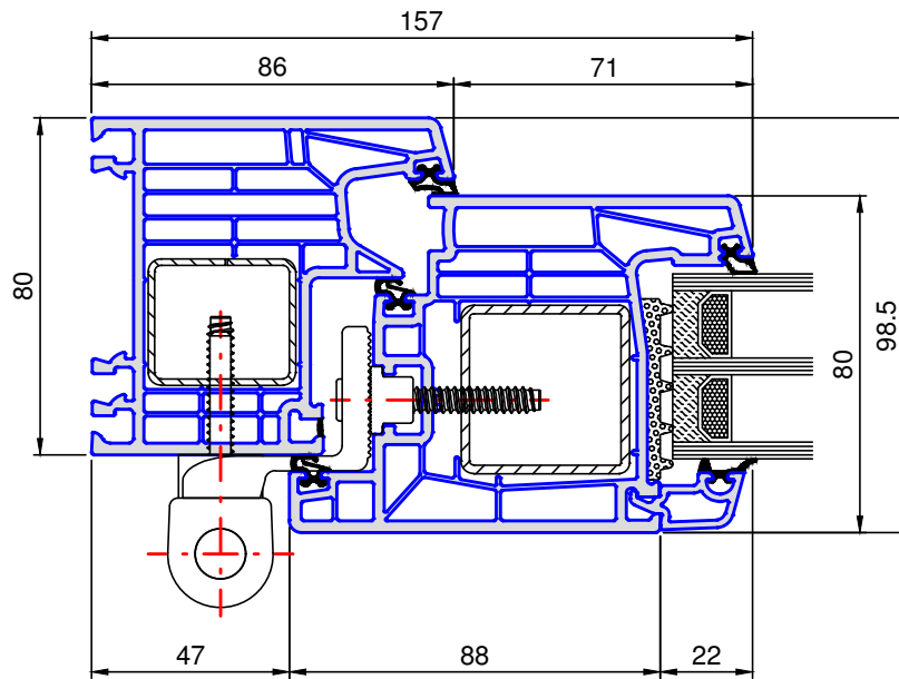
Schnitt A-A
