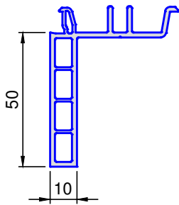
7274 .. FB-Anschluss
