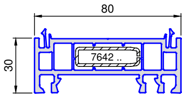
8213 .. Verbreiterung 30 / 80 mm
