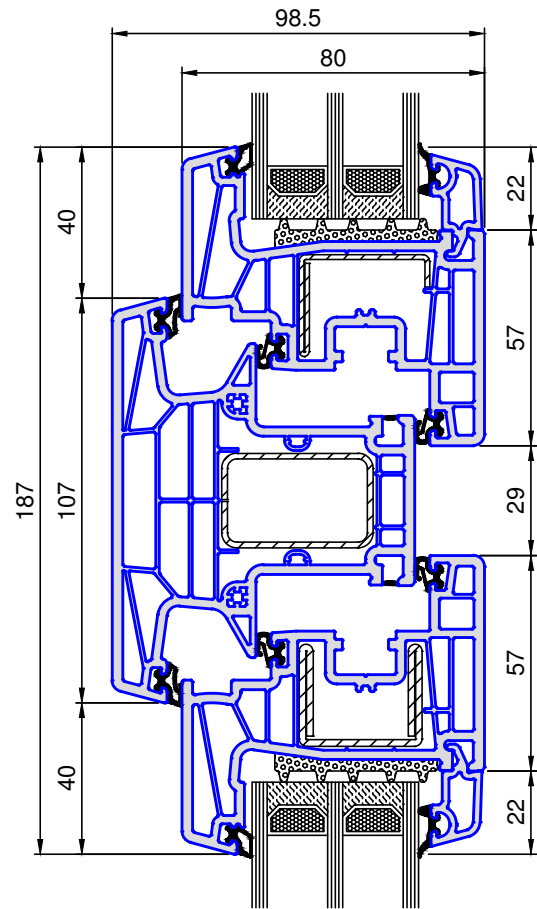
8106 .. Flügel 79
