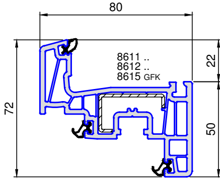
8105 .. Flügel 72 schmal
