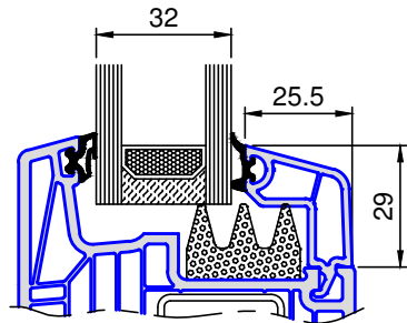
8210 .. Glasleiste Festverglasung Glas 32mm
