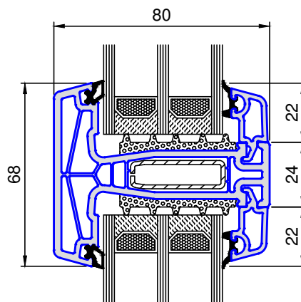
8111 .. Flügelssprosse
