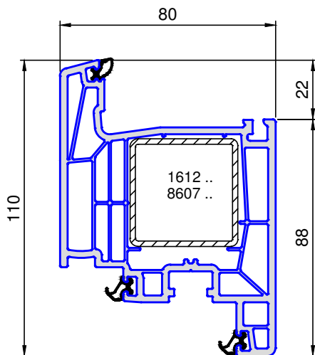
8107 .. Flügel 110
