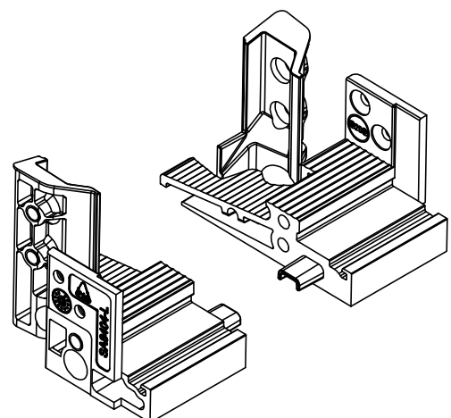
8404 .. Schwellenadapter grau mit Falz- und Schwellendichtungen
