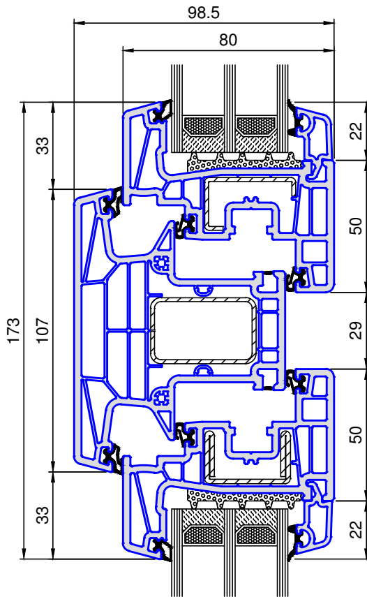
8105 .. Flügel 72 schmal
