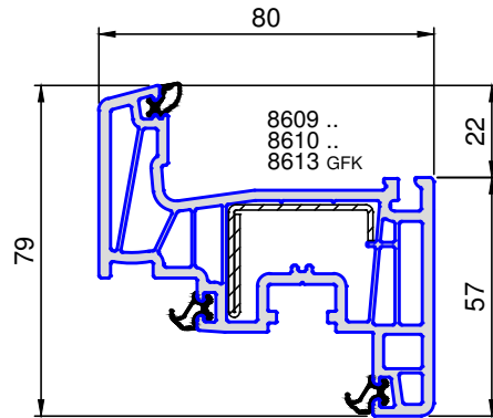
8106 .. Flügel 79
