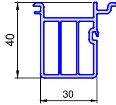
7275 .. FB-Anschlussprofil
