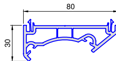
8217 .. Eckprofil variabel
