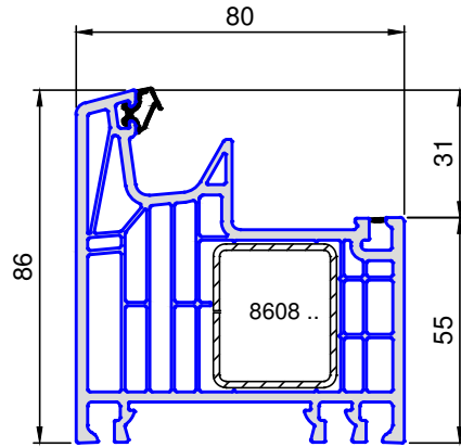
8102 .. Rahmen 86
