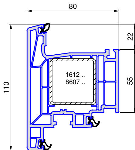
8108 .. Flügel 110 außen öffnend
