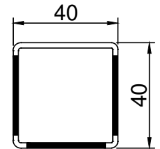
1616 .. Stahlverstärkung 40x40x2 gefräßt für Flügel 8107 und 8108
