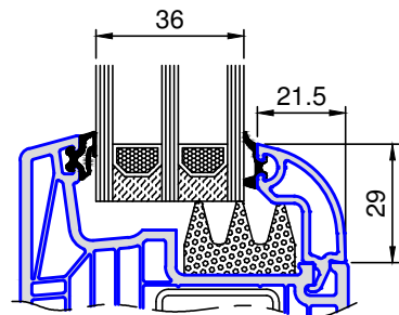
7234 .. Glasleiste Rund Festverglasung Glas 36mm
