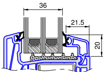
7220 .. Glasleiste Glas 36mm
