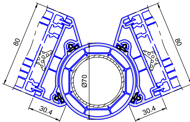
8217 .. Eckprofil variabel
