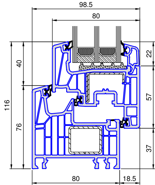
8101 .. Rahmen 76
