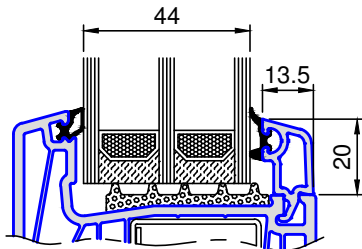
7218 .. Glasleiste Glas 44mm
