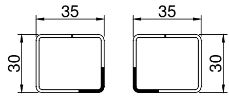
8619 .. 8620 .. Stahlverstärkung 35x30 gefräßt für Rahmen 8102
