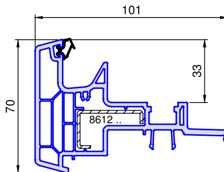
8203 .. Stulp schmal
