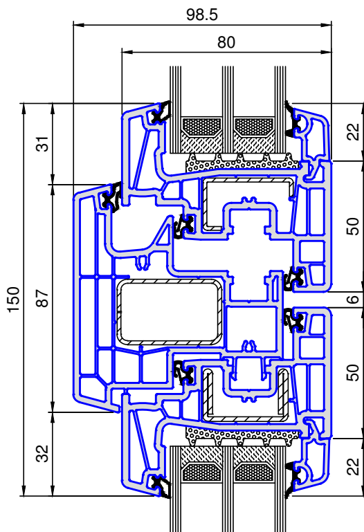
8105 .. Flügel 72 schmal
