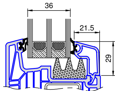
7223 .. Glasleiste Festverglasung Glas 36mm
