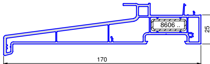
8223 .. Fensterbank 170x25
