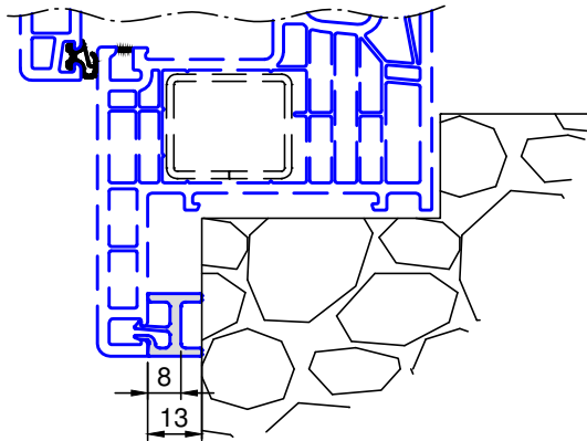
1227 .. Distanzprofil
