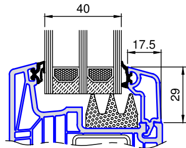
7222 .. Glasleiste Festverglasung Glas 40mm
