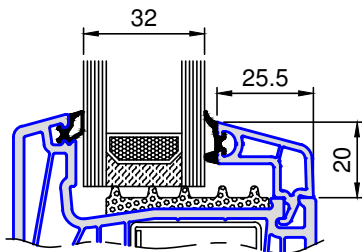
8205 .. Glasleiste Glas 32mm
