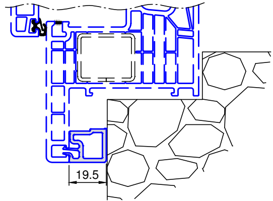
5265 .. Distanzprofil
