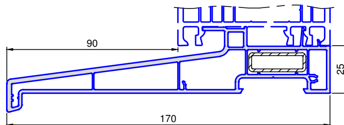
8223 .. Fensterbank 170x25
