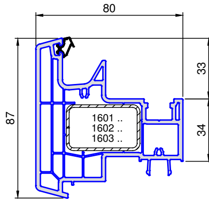
8201 .. Stulp breit
