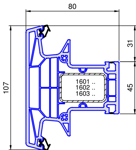
8110 .. Pfosten
