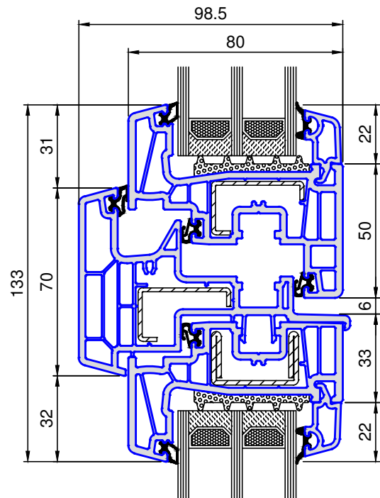
8105 .. Flügel 72 schmal
