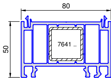
1244 .. Verbreiterung 50 / 80 mm
