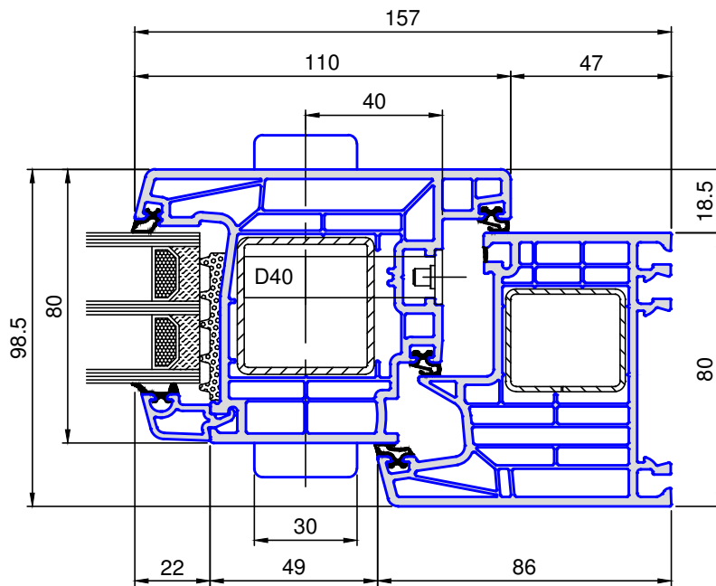
Schnitt B-B
