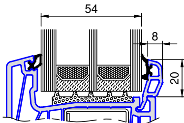
7230 .. Glasleiste Glas 54mm
