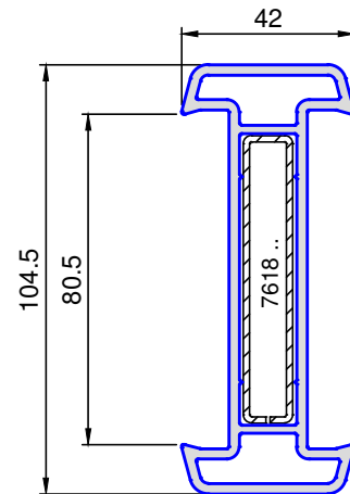
8215 .. Kopplung 80 mm
