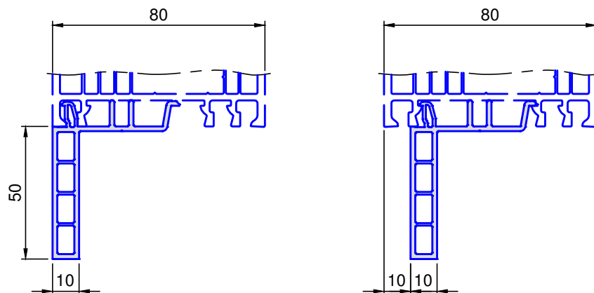
7274 .. FB-Anschluss
