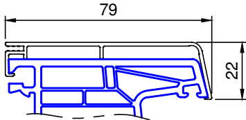
8703 .. Dualschale Rahmen 76
