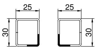
8621 .. 8622 .. Stahlverstärkung 25x30 gefräßt für Rahmen 8101
