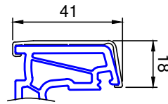
8702 .. Dualschale Flügel 72 schmal
