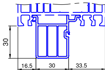
7275 .. FB-Anschlussprofil
