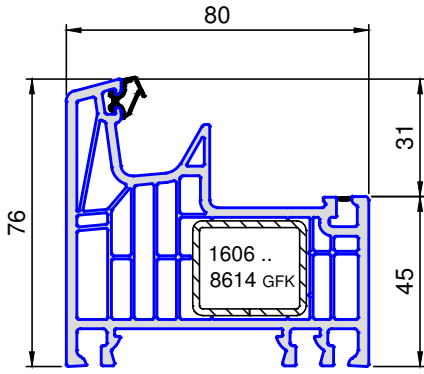
8101 .. Rahmen 76
