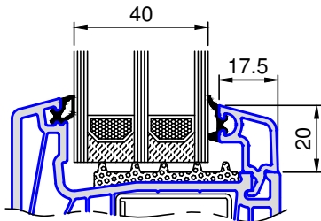
7219 .. Glasleiste Glas 40mm
