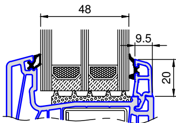
7217 .. Glasleiste Glas 48mm
