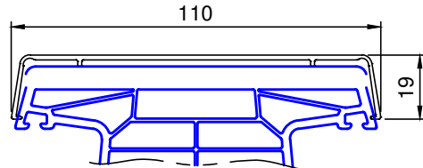
8704 .. Dualschale Pfosten
