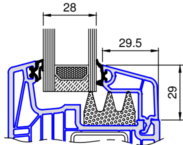
8211 .. Glasleiste Festverglasung Glas 28mm
