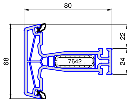
8111 .. Flügelprosse
