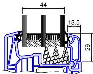
8209 .. Glasleiste Festverglasung Glas 44mm
