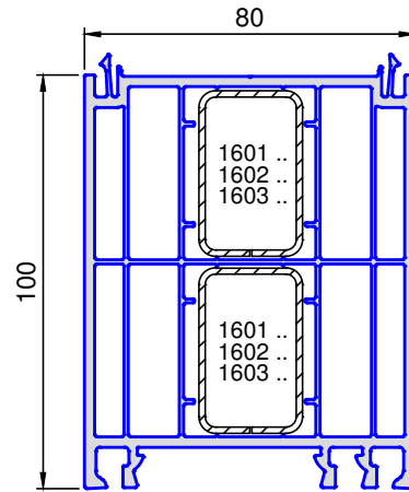
8214 .. Verbreiterung 100 / 80 mm
