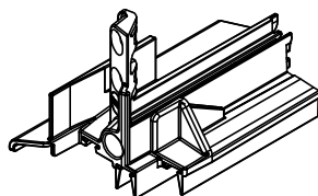
8407 .. Stulpendkappen Wetterschenkel grau rechts
