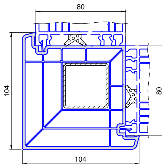
8216 .. Eckprofil 80 mm
