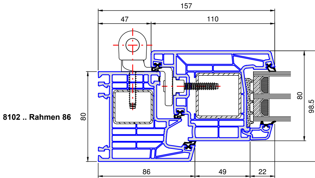
Schnitt A-A
