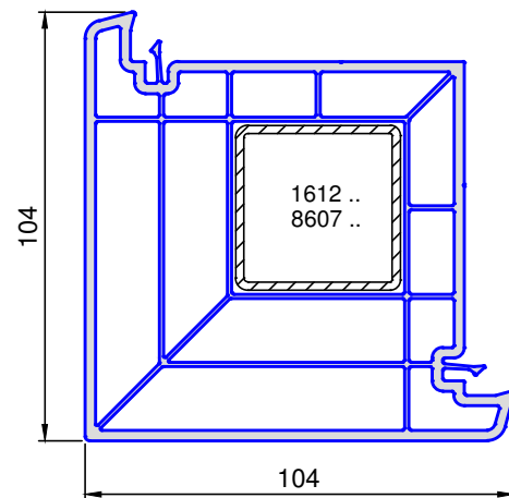
8216 .. Eckprofil 80 mm
