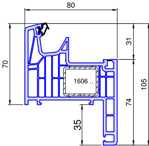
8113 .. Rahmen mit Anschlag
