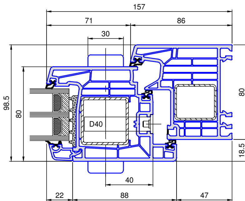
Schnitt B-B
