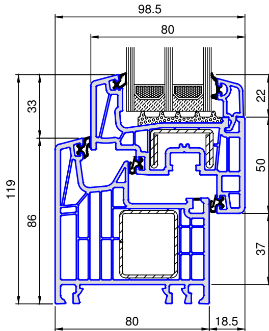
8102 .. Rahmen 86
