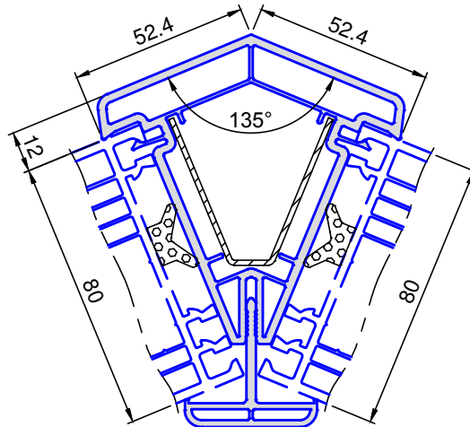
7208 .. Eckprofil 135°
